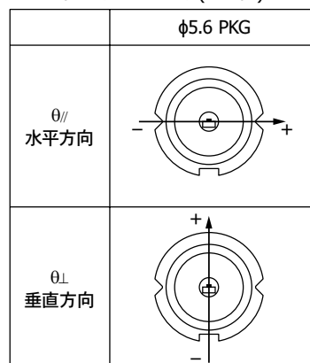
パッケージに対する FFP水平方向、垂直方向 (正面図)
