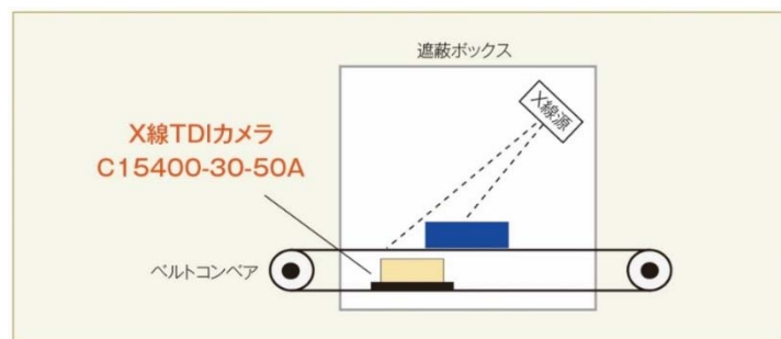
本製品によるX線非破壊検査のイメージ
